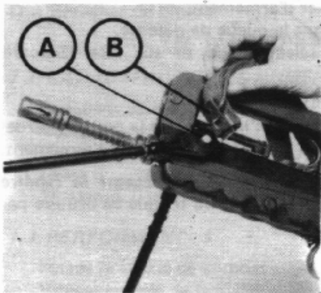
Fig. 2 - Pose du dispositif d'accrochage de la bretelle.
