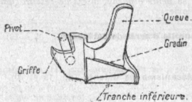
Fig. 16. — Butoir d'auget.
