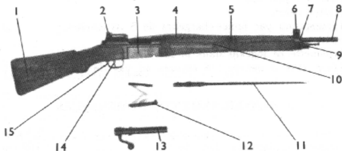
Fig. 1. — Fusil de 7,5 mm modèle 1936 (démonté).
