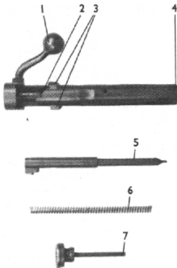
Fig. 2. — Culasse mobile (démontée).
