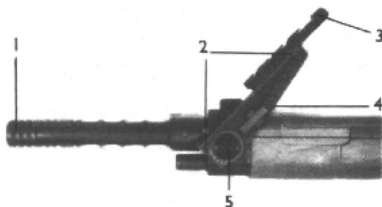
Fig. 7. — Fusil de 7,5 mm modèle 1936-1951.
