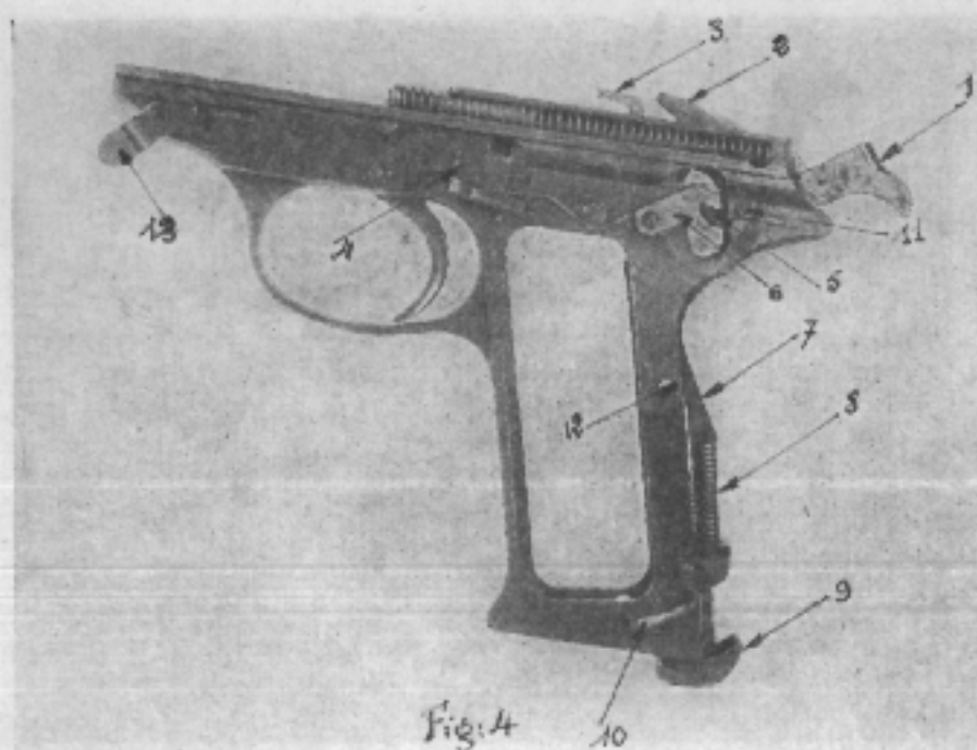
Figure 4. — La carcasse (vue du côté gauche)
