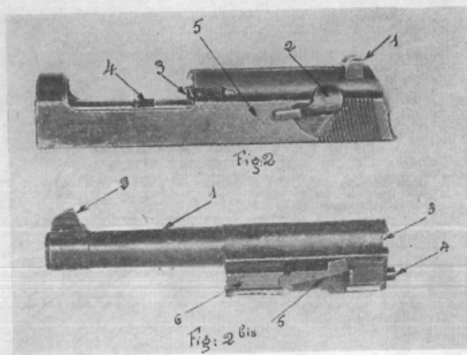
Figure 2 bis : Le canon
