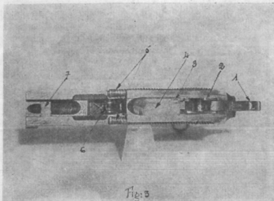
Figure 3. — La carcasse (vue de dessus)
