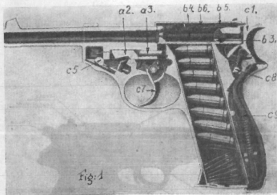
Figure 1. — Vue en coupe
