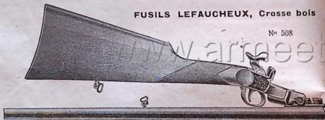
Crosse bois, fermeture à poussoir sur le côté
